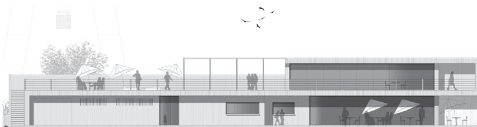
Ansicht Ost projektiertes Hafengebäude
